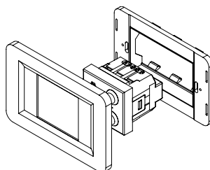
Figure 2: Montage Rectangulaire + Monture
